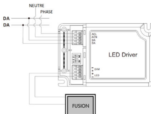
Montage pour contrôle DALI
