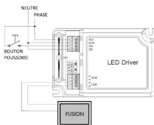
Montage gradation par bouton poussoir
